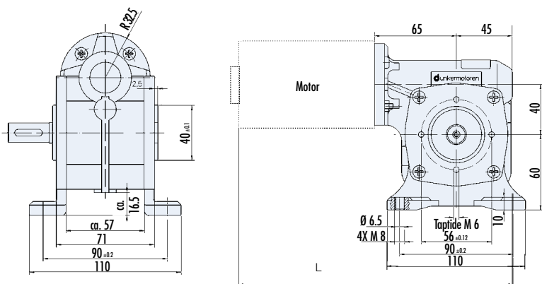
Dimensions in mm SG 120/ Maßzeichnung in mm SG 120
